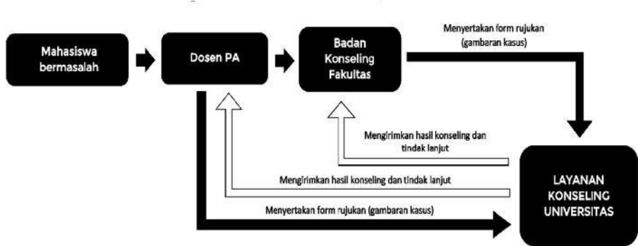
Gambar 17. Alur Rujukan
